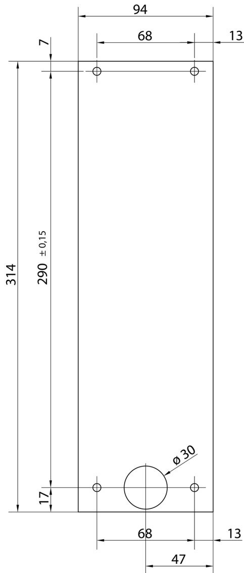
Position des orifices de montage
