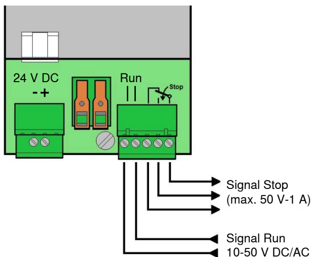
Connexion appareil de commande / machine à tisser
