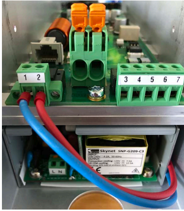
Connexions CUT-iT Dornier
