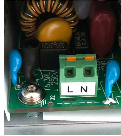
Bornes de raccordement principales 120 V AC / 240 V AC
